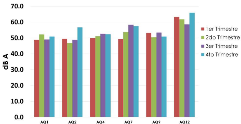
Gráfica 2. Resultados presión sonora Nivel de Presión Sonora - Período 24 Hrs
